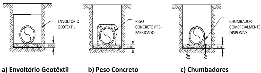
Figura 3 Alternativas de Estabilização de Tubos
